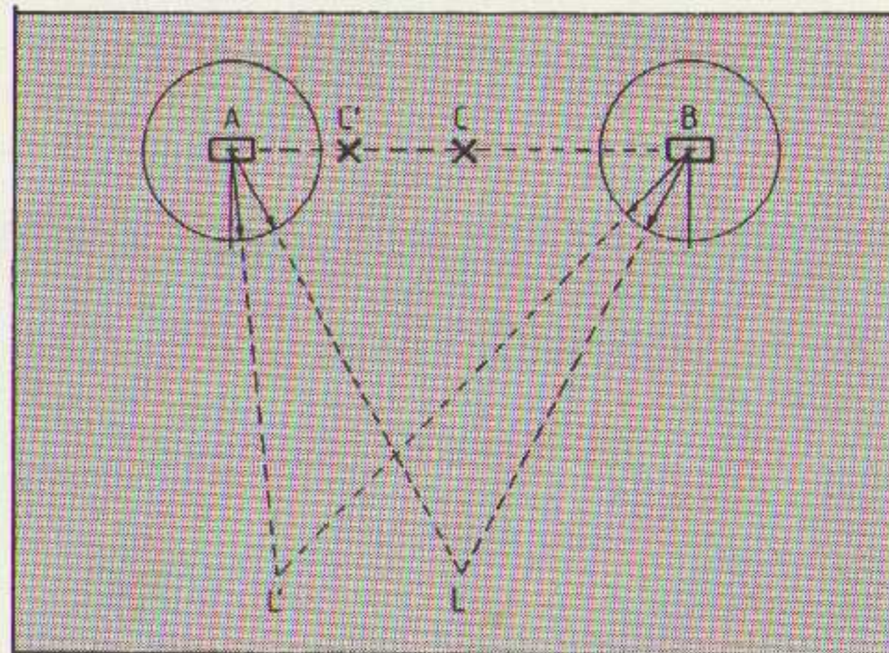
Fig. 20 Stereolokalisatie bij rondstralers.
